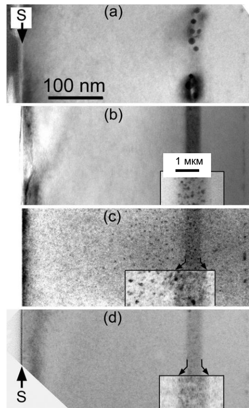
Рис. 1. Х-ПЭМ микрофотографии слоев Si/SiSn/Si после МЛЭ, имплантации C + (b-d) и отжига при 900 °C. (a) – без имплантации, (b) – 2·10 14 см -2 при 525 °C, (c) – 2·10 15 см -2 при 525 °C и (d) – 2·10 15 см -2 при RT.
