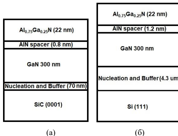
Рис. 1. Дизайн гетероструктур AlGaN/GaN: а – на SiC подложке; б – на Si подложке
