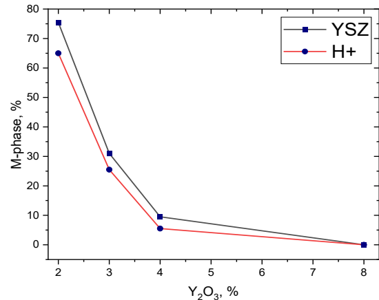
Рис. 1. Содержание моноклинной модификации в порошках диоксида циркония до и после облучения
