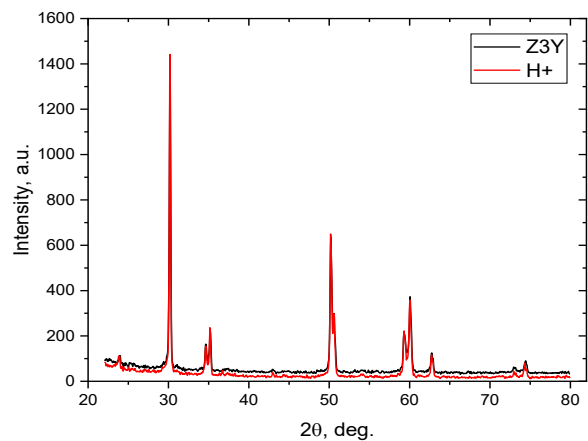
Рис. 2. Дифрактограммы керамических образцов \text{ZrO}_2 + 3 \text{mol. Y}_2\text{O}_3 до (черный) и после (красный) облучения
