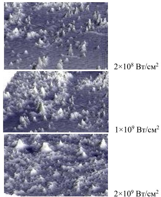
Рис. 1. 3D АСМ-изображения наночастиц Ni
