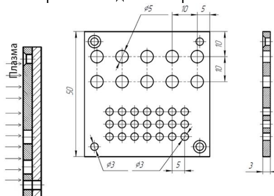
Рис. 1. Система маска-подложка
