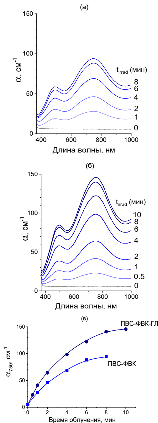
Рис. 1. Спектры коэффициента поглощения ( \alpha ) пленок ПВС-ФВК (а) и ПВС-ФВК-ГЛ (б) (33% ГЛ) до и после их УФ облучения в течение заданного времени; зависимость \alpha в максимуме при 750 нм ( \alpha_{750} ) от времени облучения пленок (в)
