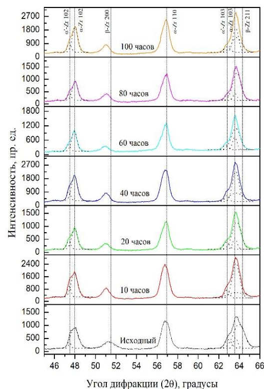
Рис. 1. Участки рентгеновских дифрактограмм образцов сплава Zr-Nb-Cr до и после отжига при температуре 350 °С: а – при угле дифракции 20-44 °; б – при угле дифракции 45-66 °
