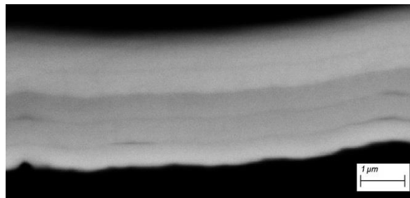
Рис. 1. Морфология поперечного сечения образца с покрытием (Zr,Hf)N/(Zr,Nb)N
